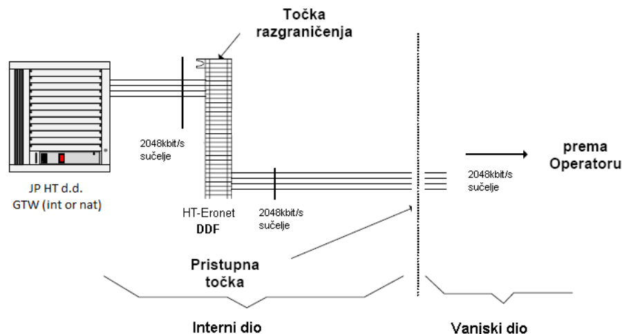
Slika 4.1.1 JP HT d.d. Mostar arhitektura međusobnog povezivanja
